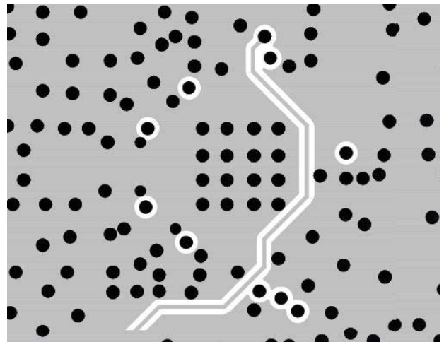
Inner Layer 3
