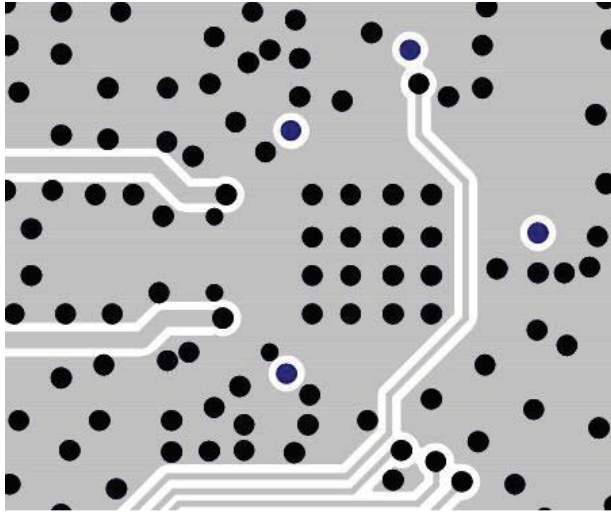
Inner Layer 4
