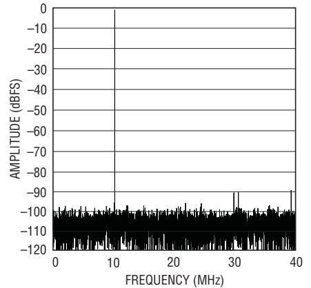
LTC2266-12: 8k Point FFT, f_{IN} = 70\text{MHz} , -1\text{dBFS} , 80\text{Mps}
