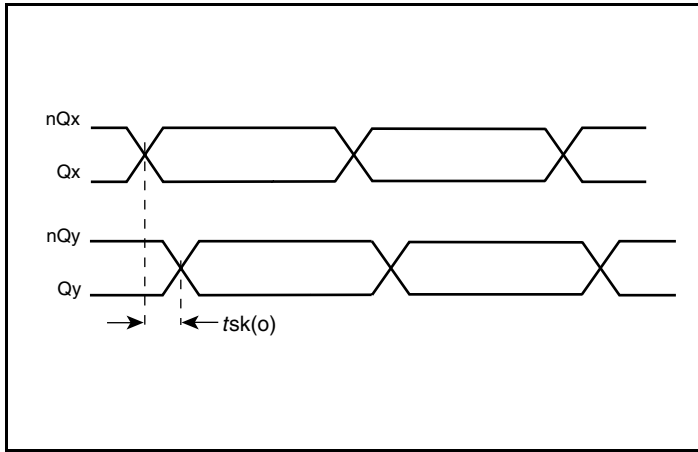
Output Skew
