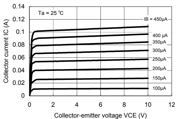
IC - VCE
