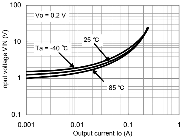
VIN - Io
