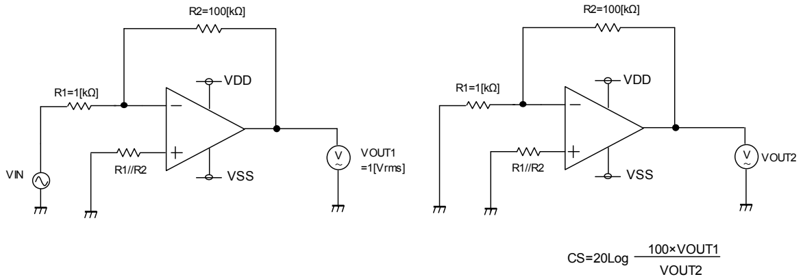
Fig. 189. Test circuit3
