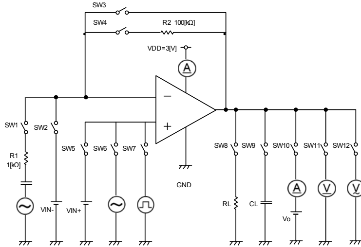
Fig. 186. Test circuit2
